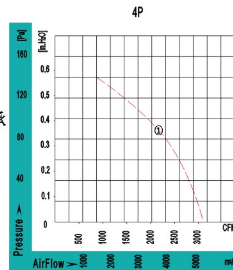
Ø420-5 137系列轴流风机 Ø420-5 137Series Axial Fan
